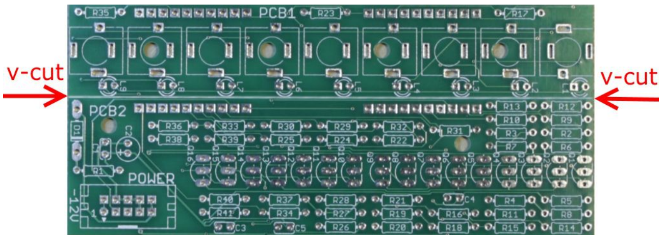
Empty PCB.
